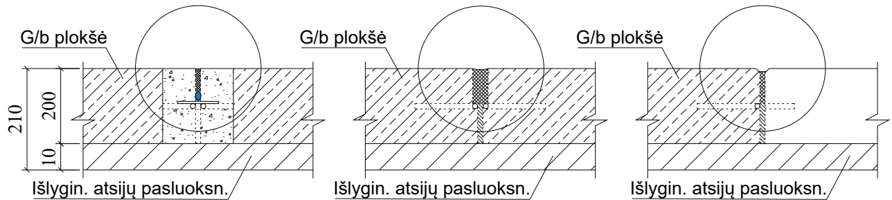
Pjūvis 2-2
